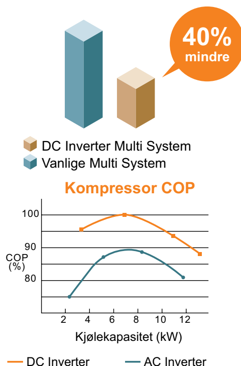
DC Twin Rotasjons kompressor
